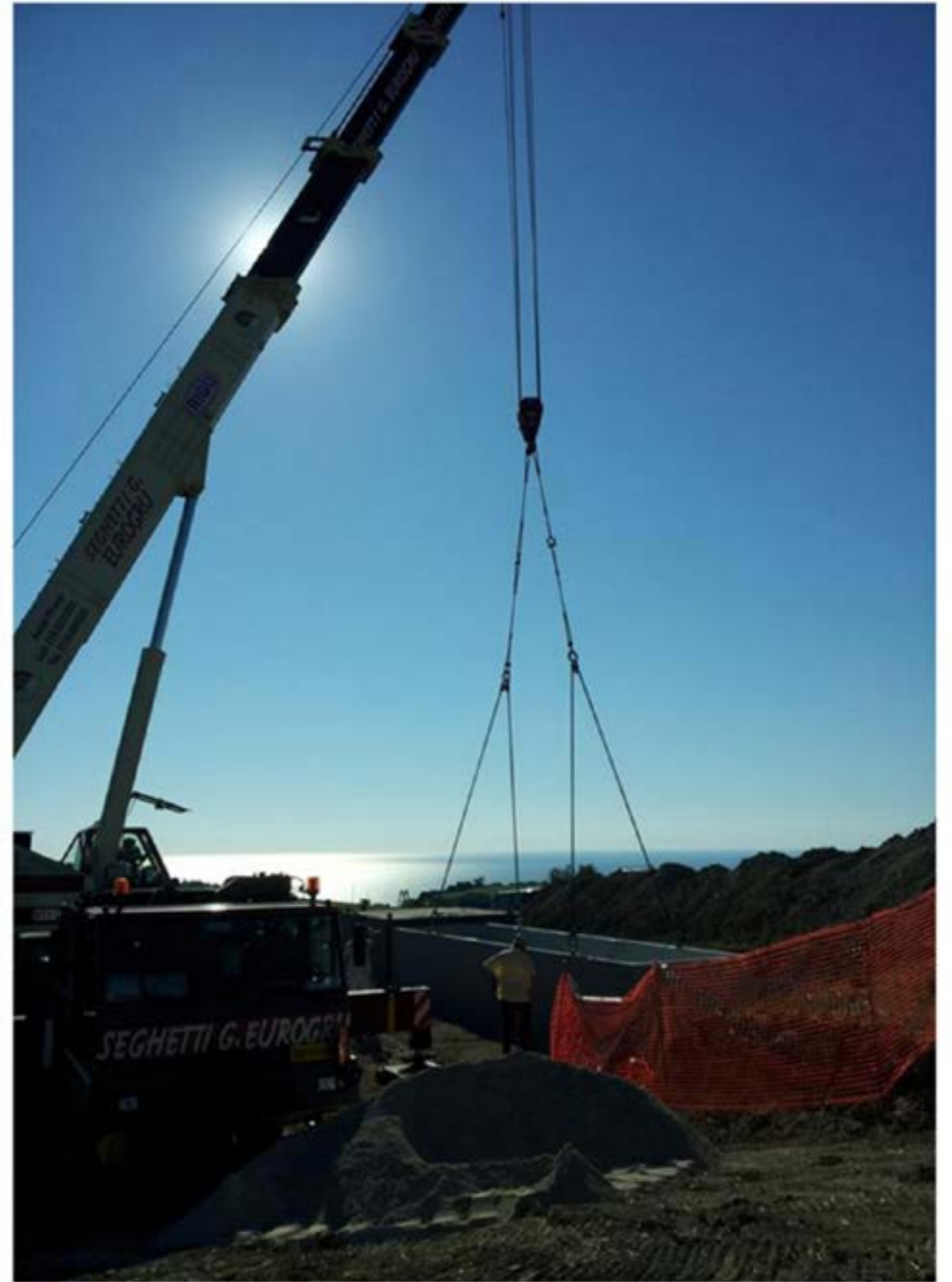
Autogru T.120 - Sollevamento Vasca in cemento
